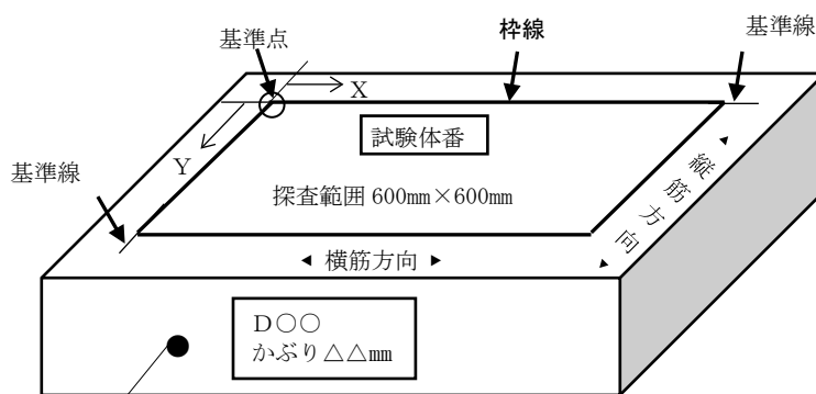
比誘電率の設定に使用する鉄筋 (いずれかの側面に●シールで示す)
